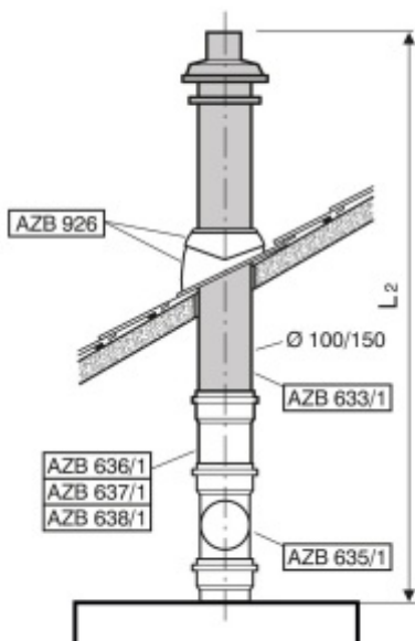
Svislé přes šikmou střechu
