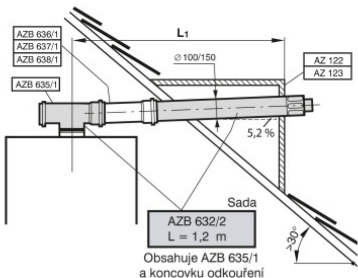
Vodorovně přes šikmou střechu, případně skrz stěnu (pozor na ustanovení ČSN 73 4201)
