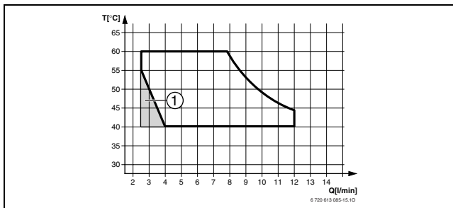
Obr. 11 Graf pro vstupní teplotu studené vody +15 °C (ZWC 24-3 MFA/MFK)
